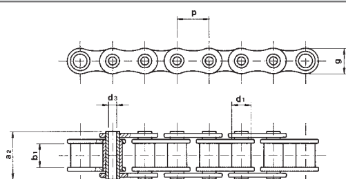
Typ A - Łańcuchy tulejkowe
